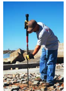
Fonçage manuel avec le marteau guidé
