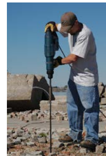
Fonçage motorisé avec le perforateur GBH11-DE
